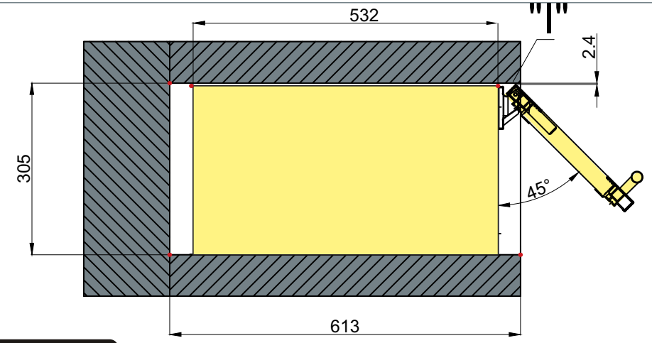
ВИД СВЕРХУ
