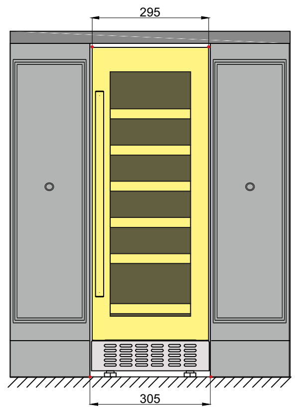
ВИД СПЕРЕДИ
